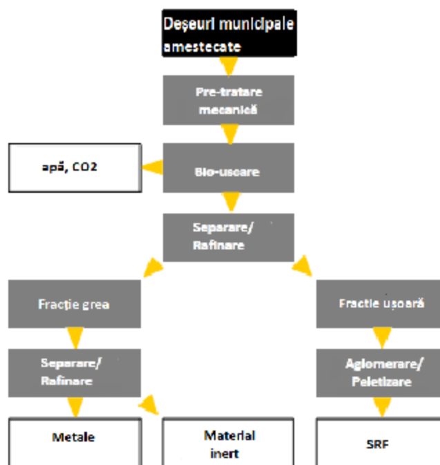
Figura 7-17 TMB cu biouiscare – schema fluxului
