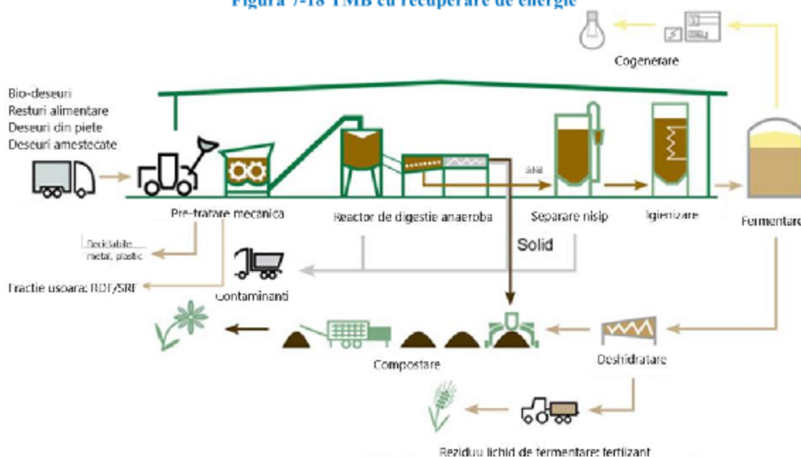
Figura 7-18 TMB cu recuperare de energie
